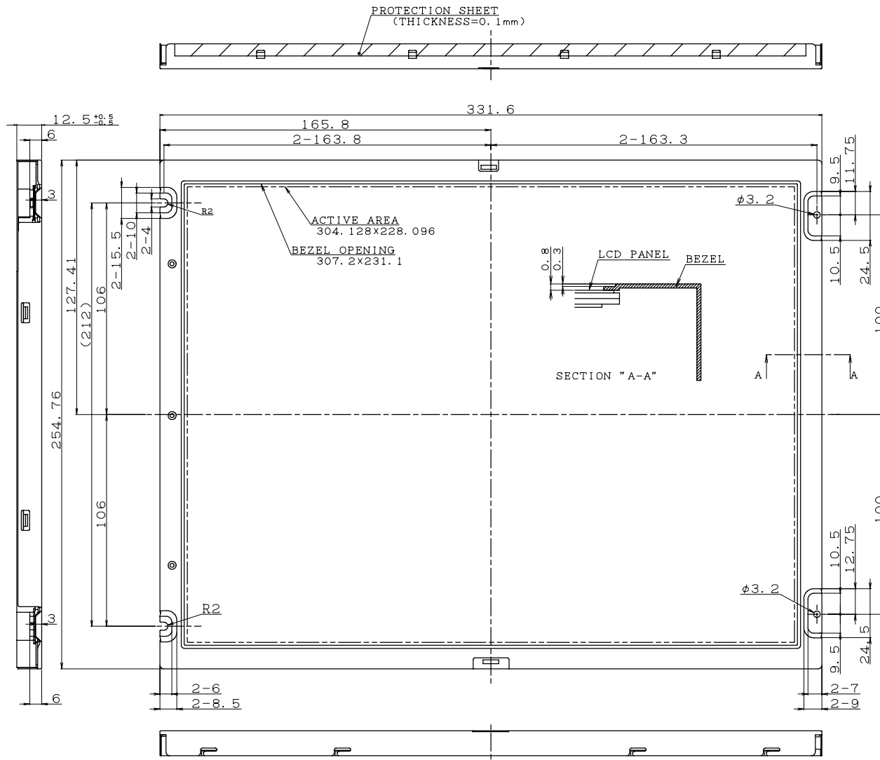
BEZEL/DISPLAY POSITION
